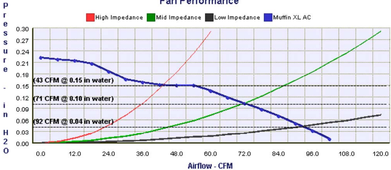
Fan Performance
